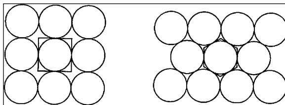
Configuraciones de círculos (cuadrada y hexagonal).
